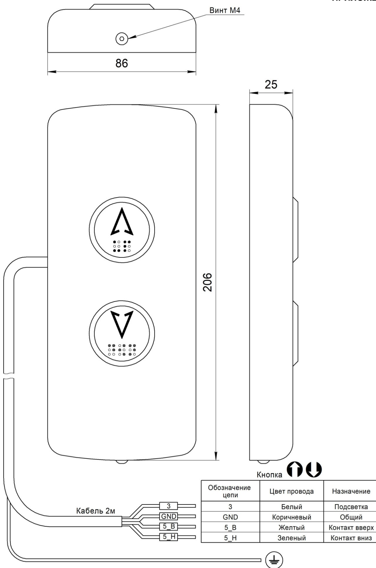
Рис.1 Внешний вид, габаритные и установочные размеры Вызывного поста ВП-2103-05
